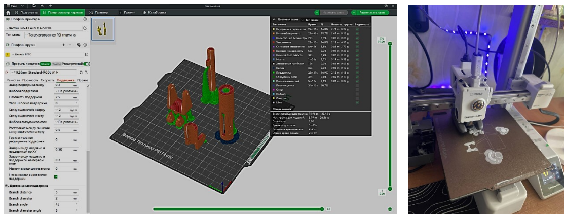
Рис.2. Етапи друку
